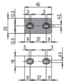
SM D•T actuator
